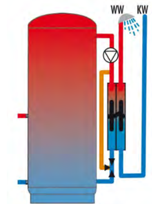
Abb.12: Systemspeicher mit Frischwassermodul
